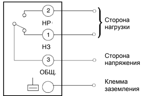
Рис. 2. Схема соединений реле С6097А
