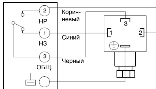
Рис. 3. Схема соединений реле С6097А с разъемом DIN
